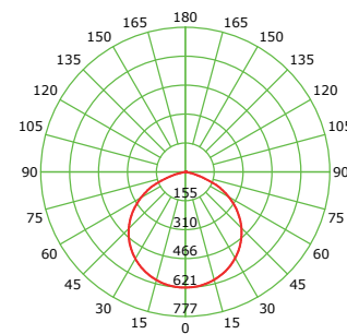
CURVA FOTOMETRICA
